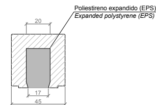
SECCIÓN B-B' / SECTION B-B'
