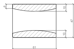
SECCIÓN A-A' / SECTION A-A'
