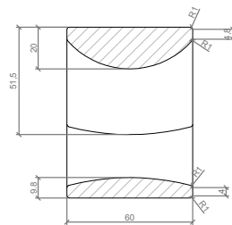
SECCIÓN A-A' / SECTION A-A'
