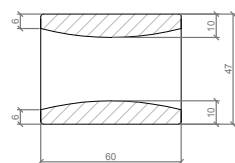
SECCIÓN A-A' / SECTION A-A'
