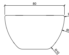
PERFIL / RIGHT SIDE
