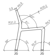
PERFIL / SIDE
