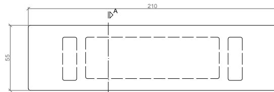
PLANTA / TOP VIEW
