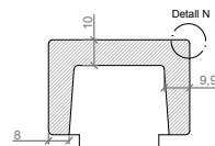
SECCIÓN / SECTION
