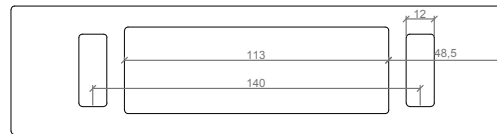
PLANTA INFERIOR / BOTTOM VIEW
