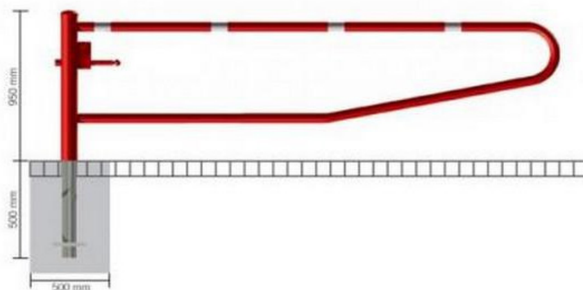
Barrière pivotante avec clé triangle
