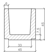
SECCIÓN B-B' / SECTION B-B'
