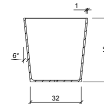
SECCIÓN A-A' / SECTION A-A'
