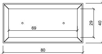
PLANTA / TOP VIEW
