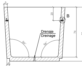
SECCIÓN A-A' / SECTION A-A'
