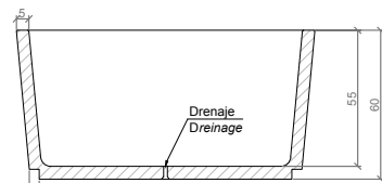
SECCIÓN A-A' / SECTION A-A'
