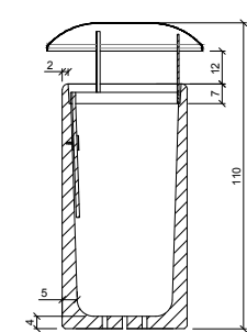
SECCIÓN A-A' / SECTION A-A'
