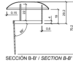
SECCIÓN B-B' / SECTION B-B'
