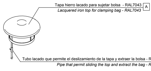
DETALLE ACCESORIO / DETAIL ACCESSORIES
