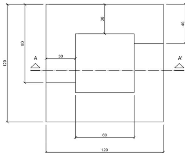
PLANTA / TOP VIEW
