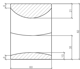
SECCIÓN A-A' / SECTION A-A'
