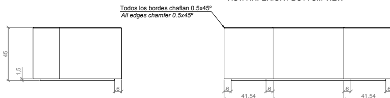
PERFIL / RIGHT SIDE
