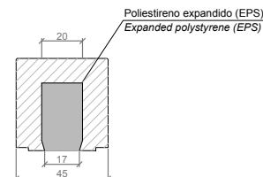
SECCIÓN B-B' / SECTION B-B'
